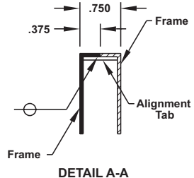
DETAIL A-A
