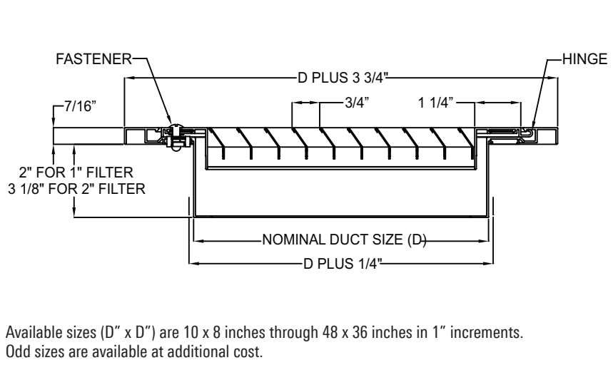
350RLF1 / 350RLF2 - Border Type 1(Surface Mount) & Border Type 3 (Lay-in T-Bar)
